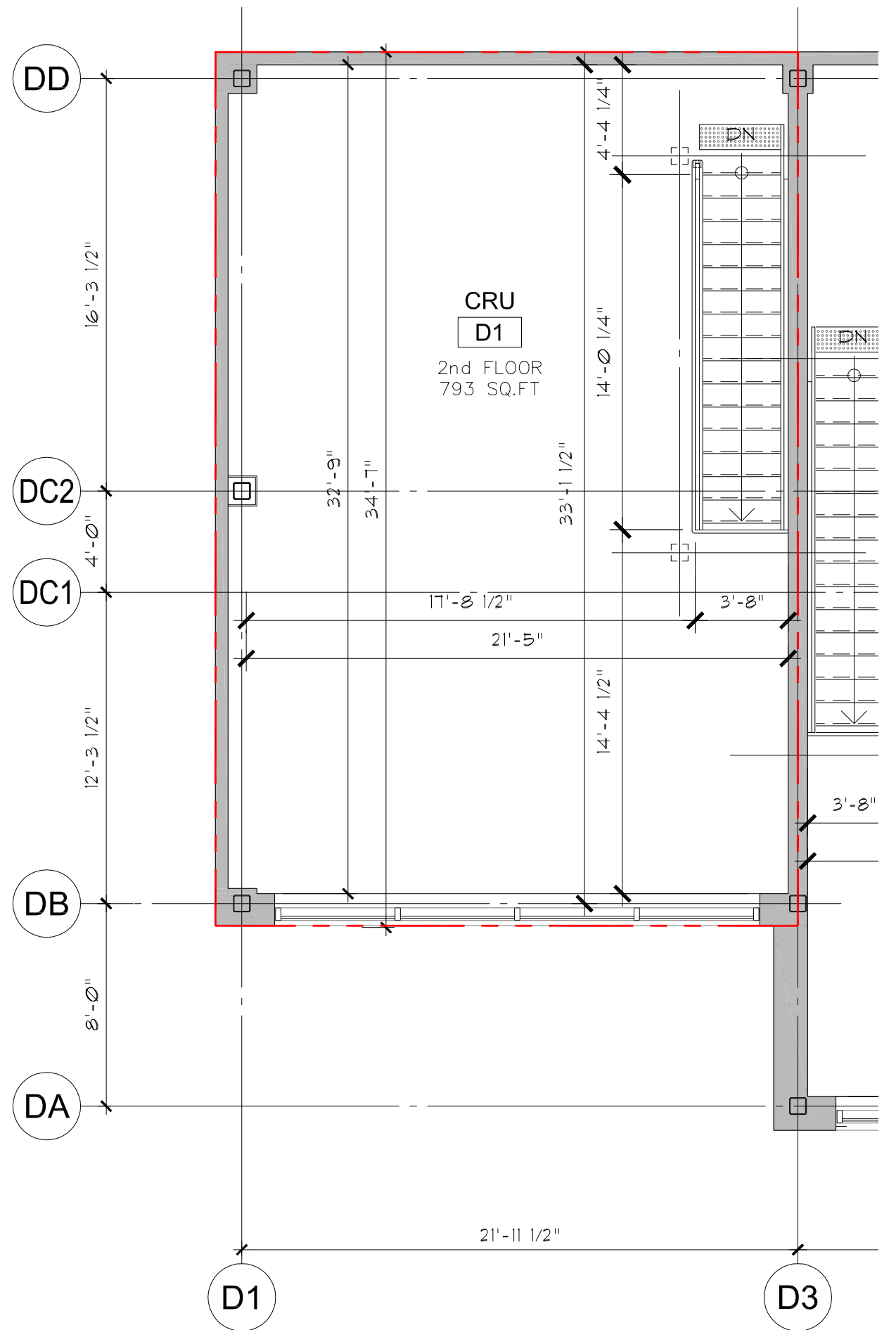
2 UNIT D1 - SECOND FLOOR SCALE: AS PER SCALE BAR
